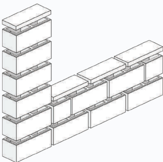
Sposób ułożenia na mijankę
